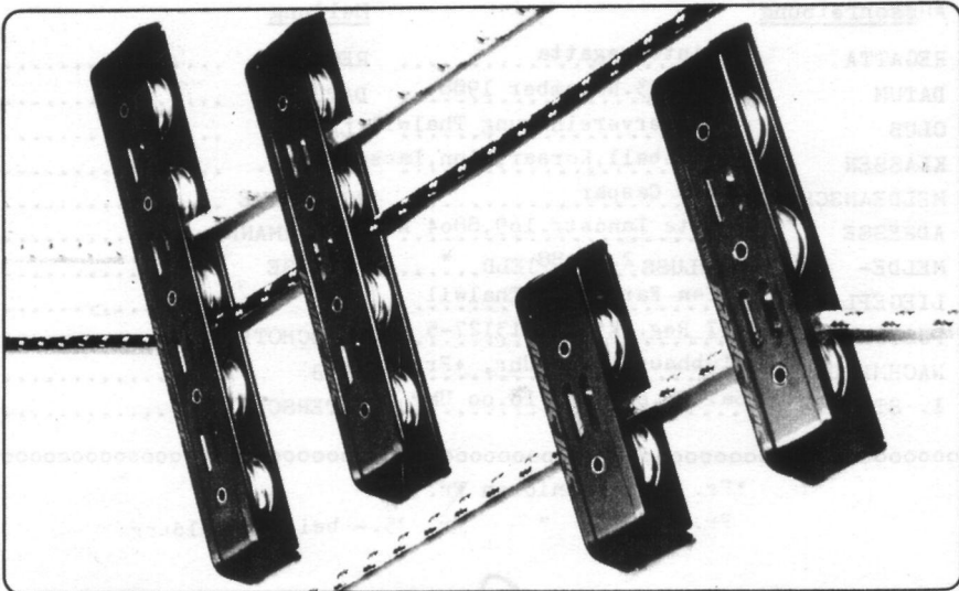
poulie violon avec ringot et serre-écoute réglable
